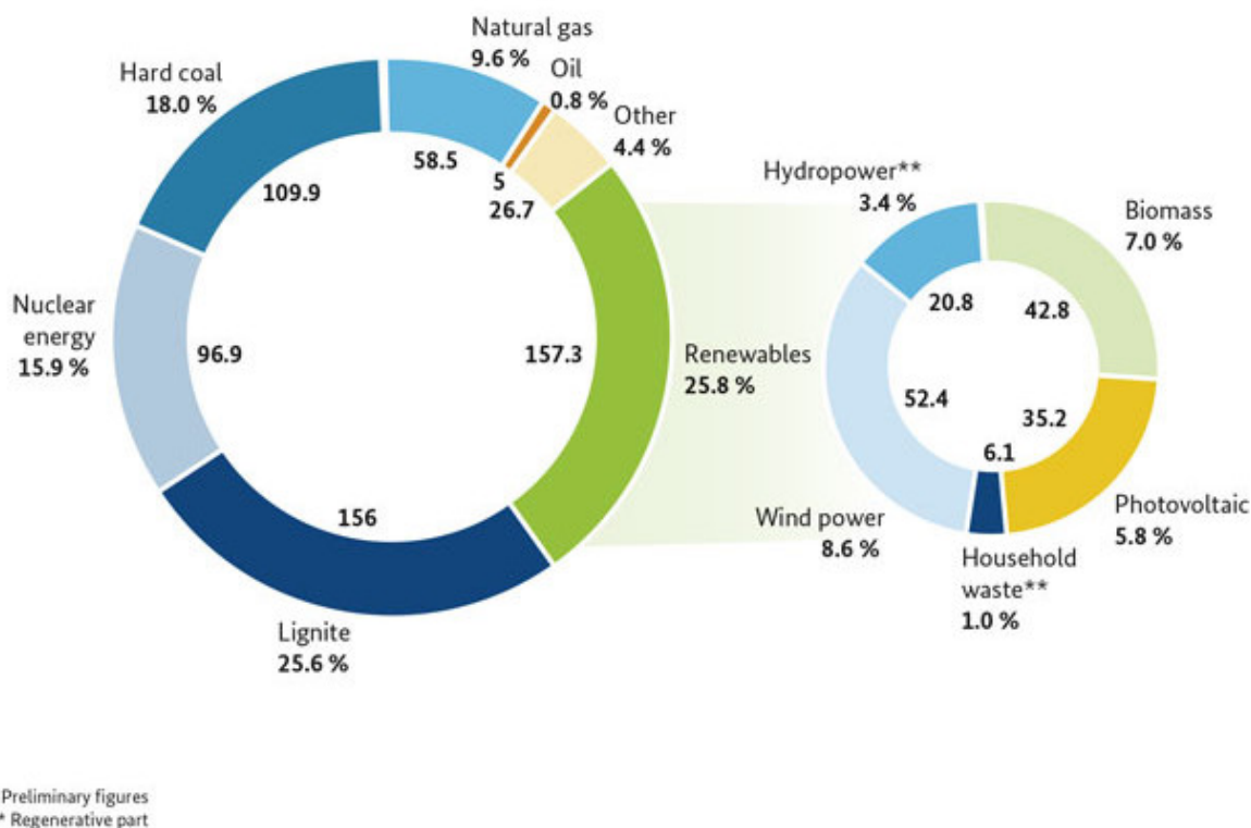
図：ドイツのエネルギー構成 (2014 年度)
